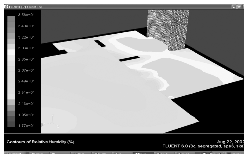
تصویر ۱۶- کانتور رطوبت در مدل ۱. (ماخذ: نگارنده)
