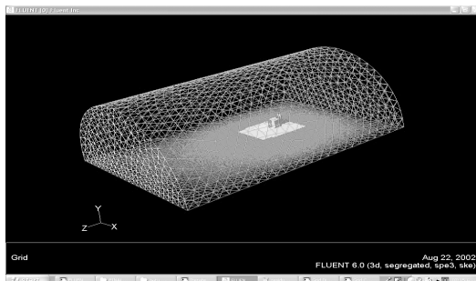
تصویر ۱۲- نمایی از هندسه خانه رسولیان در محدوده جریان. (ماخذ: نگارنده)
