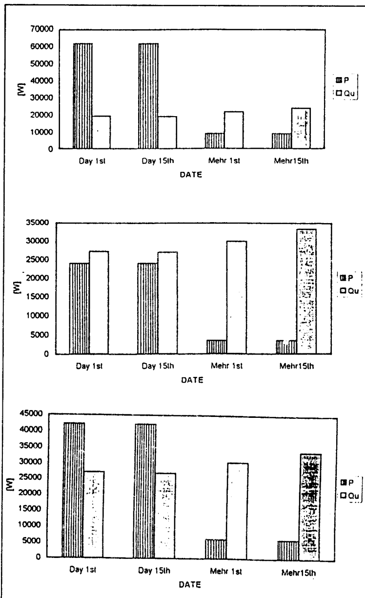
نمودار ۳. میزان نیاز حرارتی (P) و گرمای جذب شده ( Q_{II} ) برای دهانه‌های غربی (بالا، میانی (وسط)، و شرقی (پائین)).
