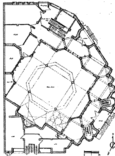
تصویر (۵): پلان همکف مسجد الرسول
